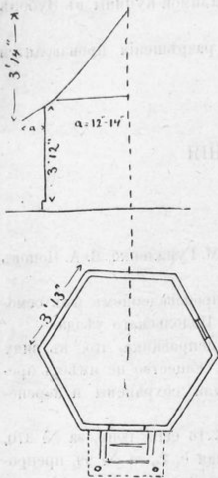
Рис. 33. Часовня при с. Поливановѣ, Подольскаго уѣзда, Моск. губ.
