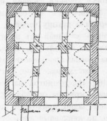
Рис. 36. Никольскій храмъ Новоспасскаго монастыря.
