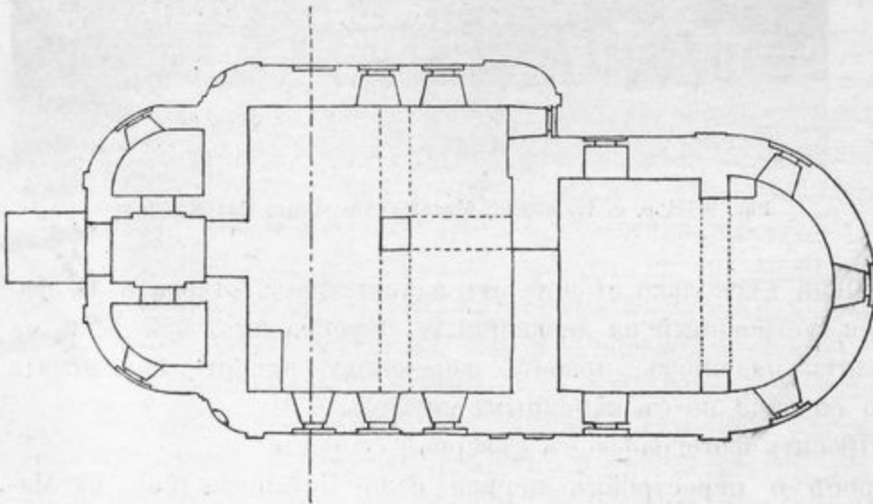
Рис. 8. Планъ церкви при Императорскомъ Тульскомъ Оружейномъ заводѣ.
