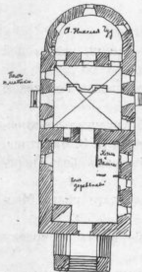
Рис. 18. Цер. с. Никольскаго-Колчева, Подольскаго уѣзда, Московской губ.
