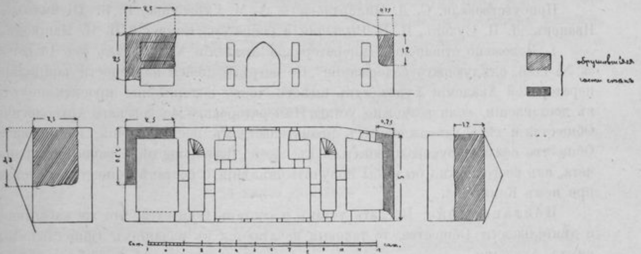
Чер. 26. Сердарскій дворецъ въ г. Эривани.
